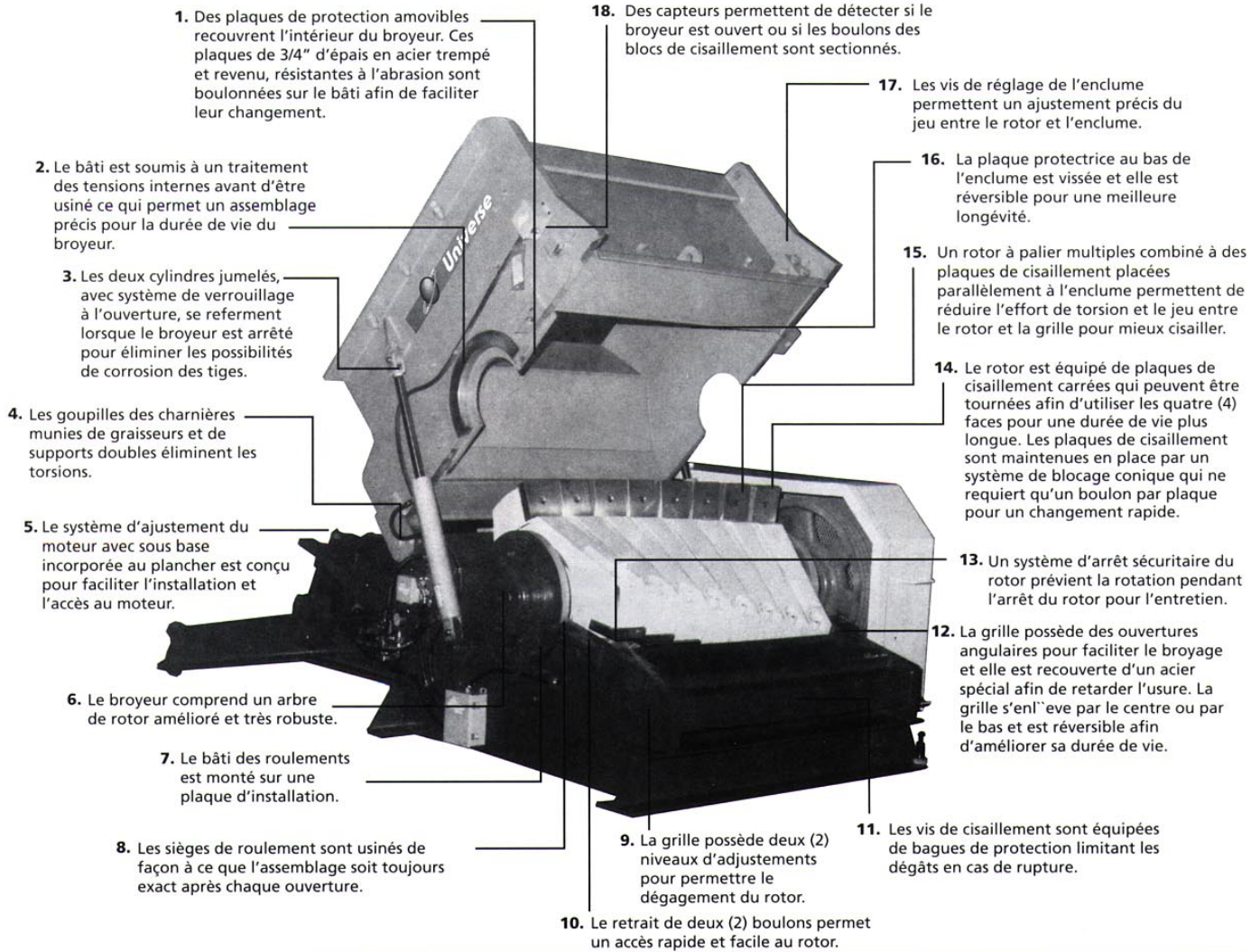
Rotor à trois (3) paliers (de série)
